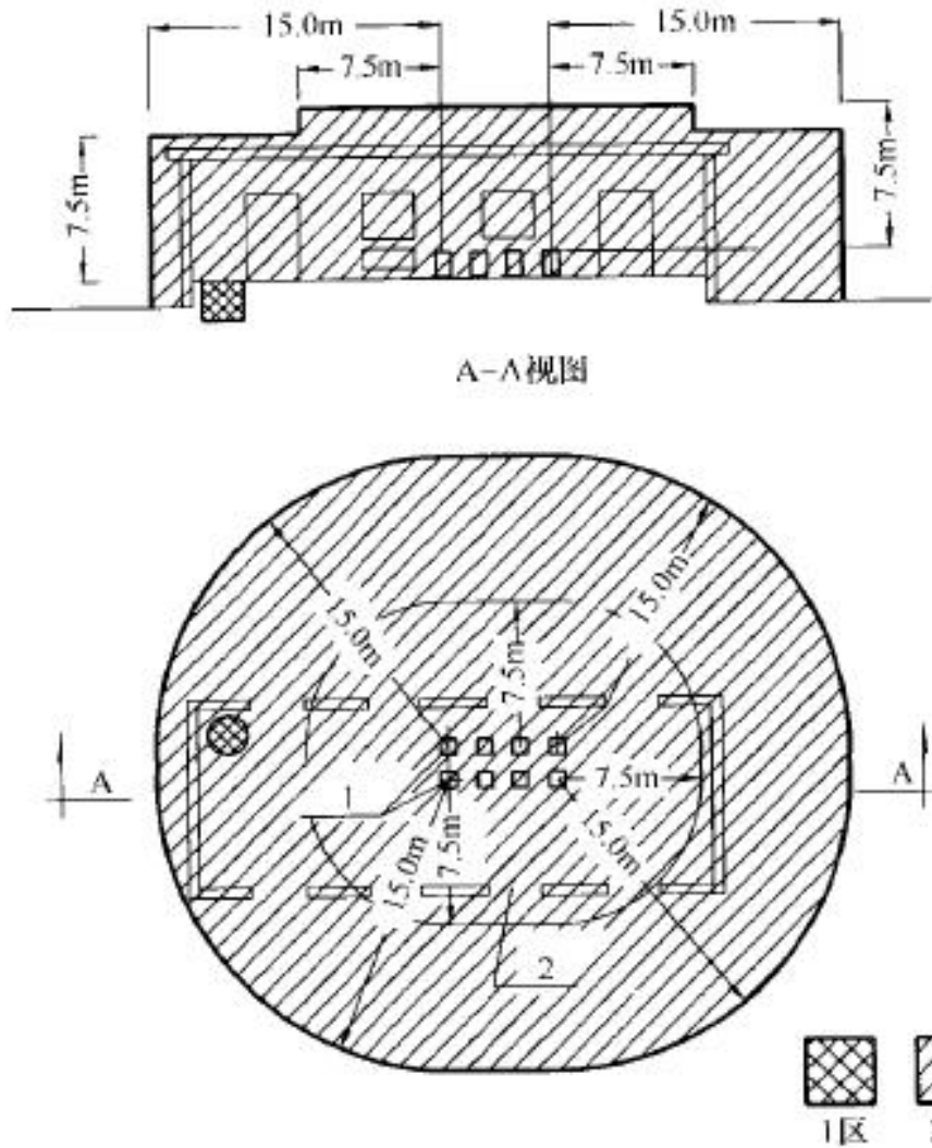
图 A.0.2 通风良好的生产性建筑爆炸危险区域等级和范围划分图
