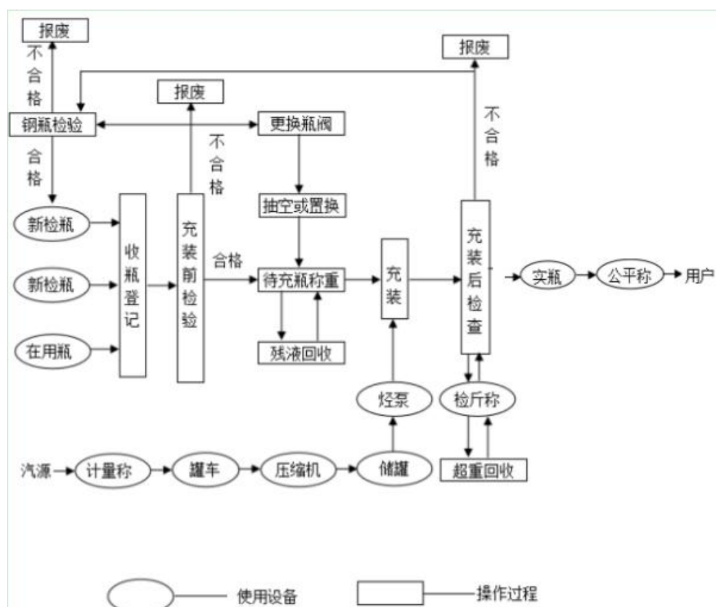
图 2.5.1-1 液化石油气气瓶充装工艺流程图
