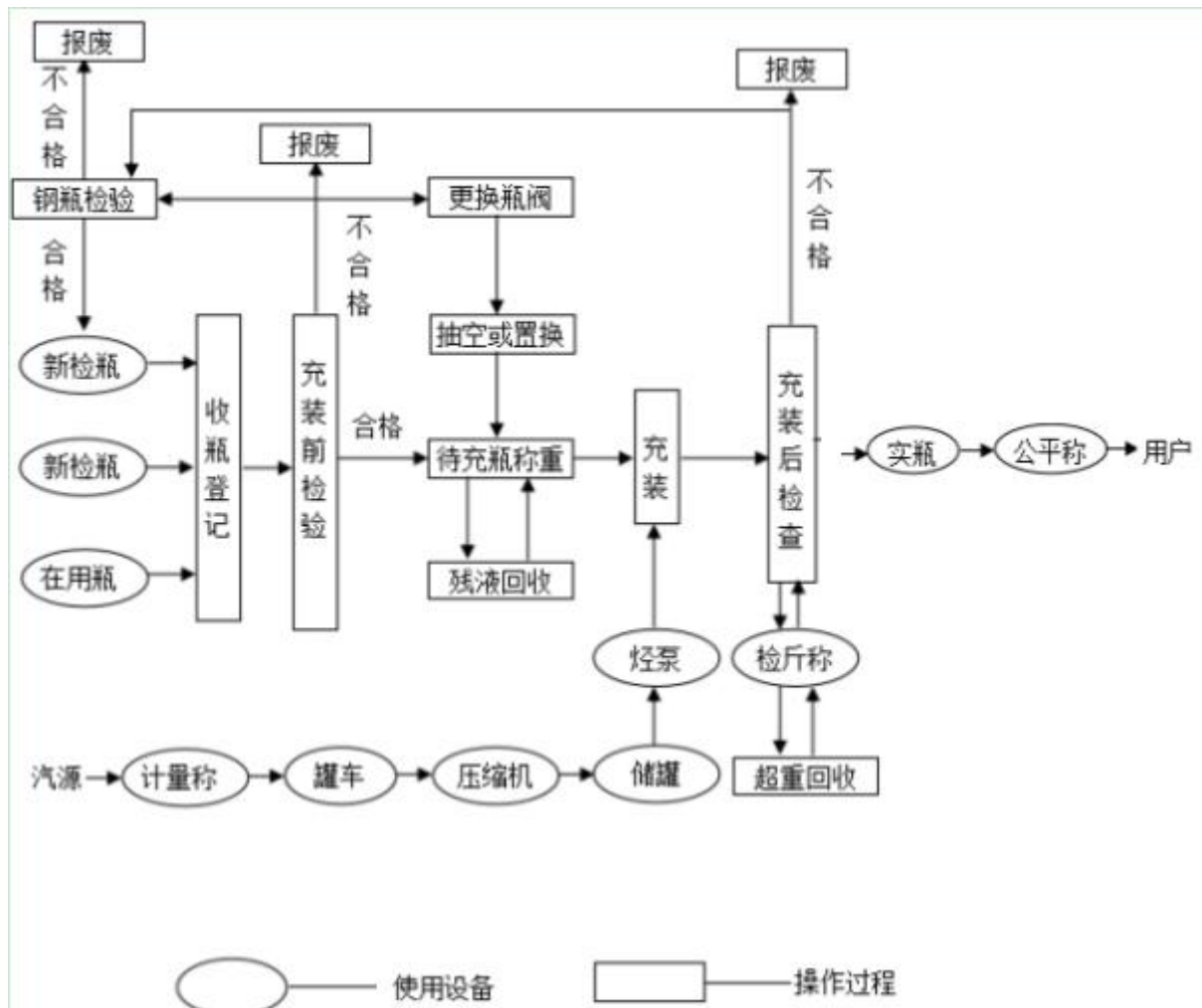
图 2.5.1-1 液化石油气气瓶充装工艺流程图
