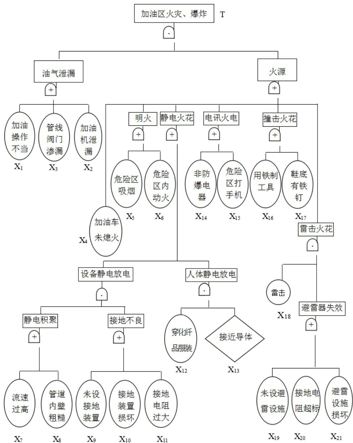
附图 4-1 加油区火灾、爆炸事故树
