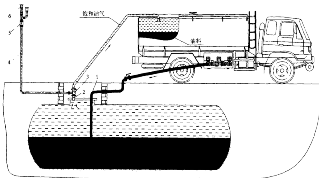
图 1 第一阶段油气回收系统示意图
