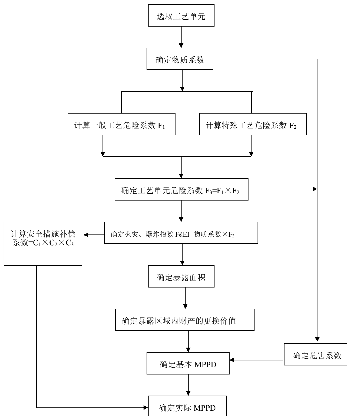
图 4.2.2-1 道七版风险分析计算程序图
