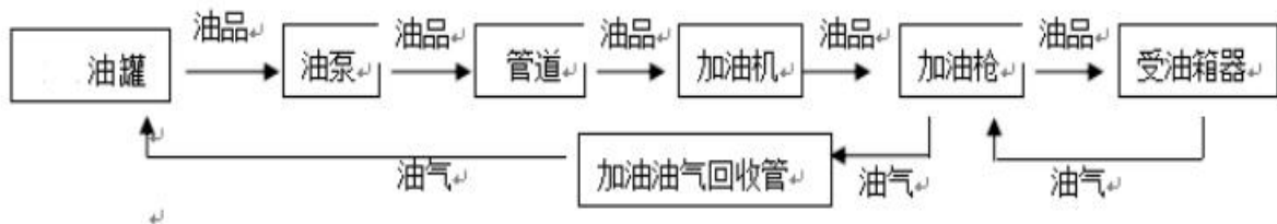
图 2.2-1 汽油加油工艺流程图
