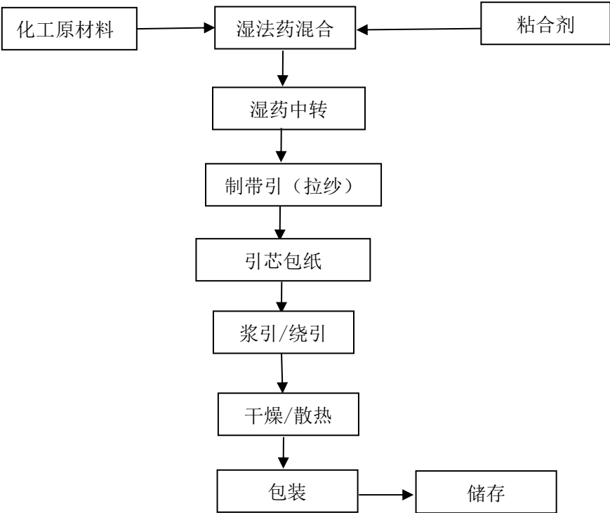
图 2-4-6 带引产品生产工艺流程图
