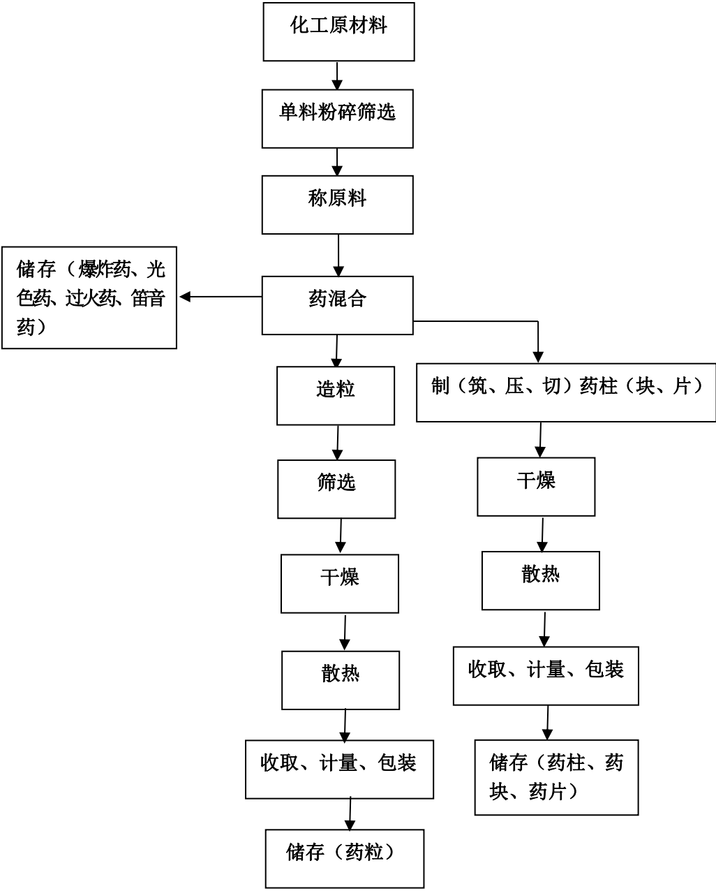
图 2-4-1 药物裸药效果件生产工艺流程图
