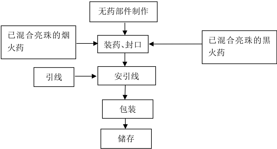
图 2-4-2 喷花类生产工艺流程图
