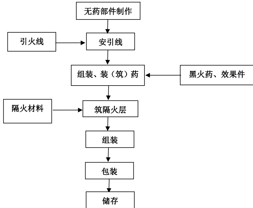
图 2-4-4 吐珠类产品生产工艺流程图
